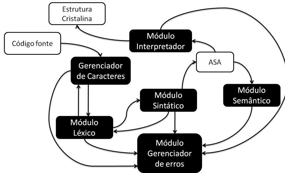
Figura 8.1: Visão Geral do Compilador.
