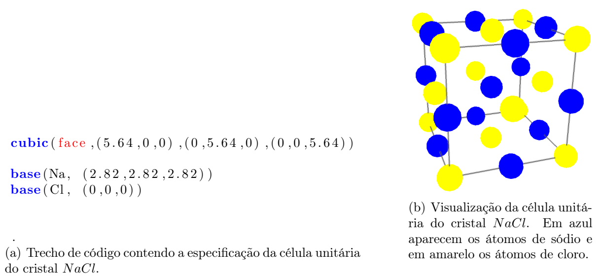
Figura 9.2: Definição da estrutura cristalina do cloreto de sódio.
