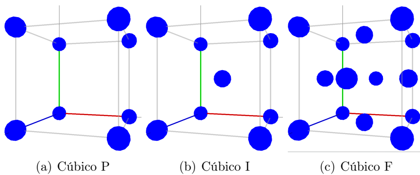
Figura 2.5: Retículos Cúbicos com os vetores que definem sua rede em destaque.
