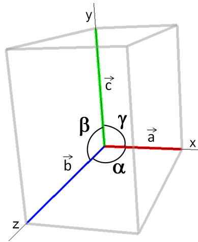
Figura 2.8: Sistema Ortorrômico.
