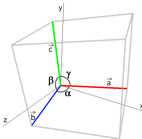
Figura 2.14: Sistema Romboédrico.
