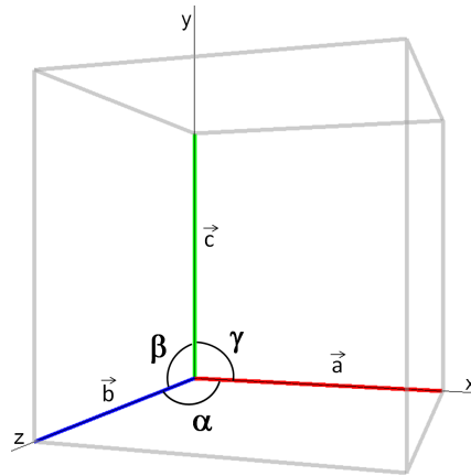
Figura 2.4: Sistema Cúbico.
